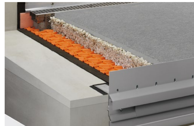
Конструкция покрытий на подстилке из гравия / щебня с Schlüter-TROBA
