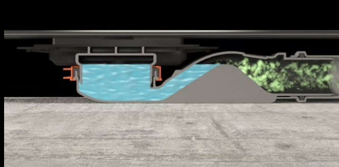
Постоянный сифонный затвор благодаря волнообразной форме
